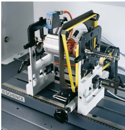
Auswuchtmaschine HM10 mit Klappbügelbandantrieb
